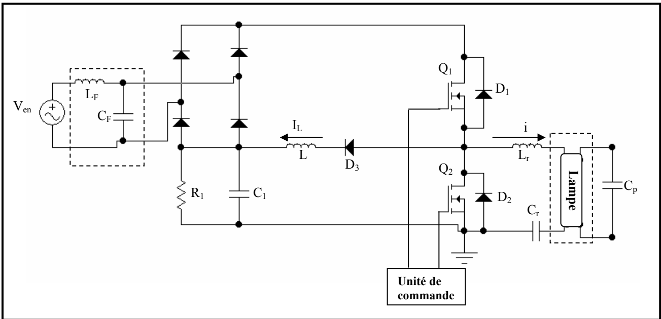
Fig.3.17 : Circuit réduit du ballast électronique
