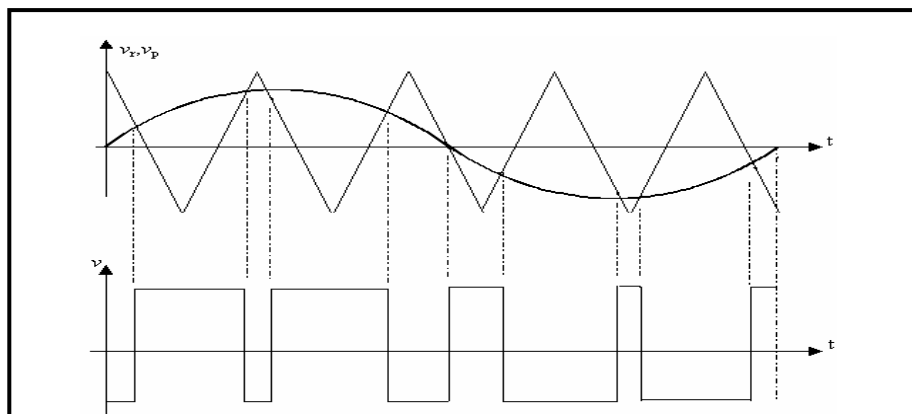
Fig.3.8.a: Sous modulation ( r < 1 ).
