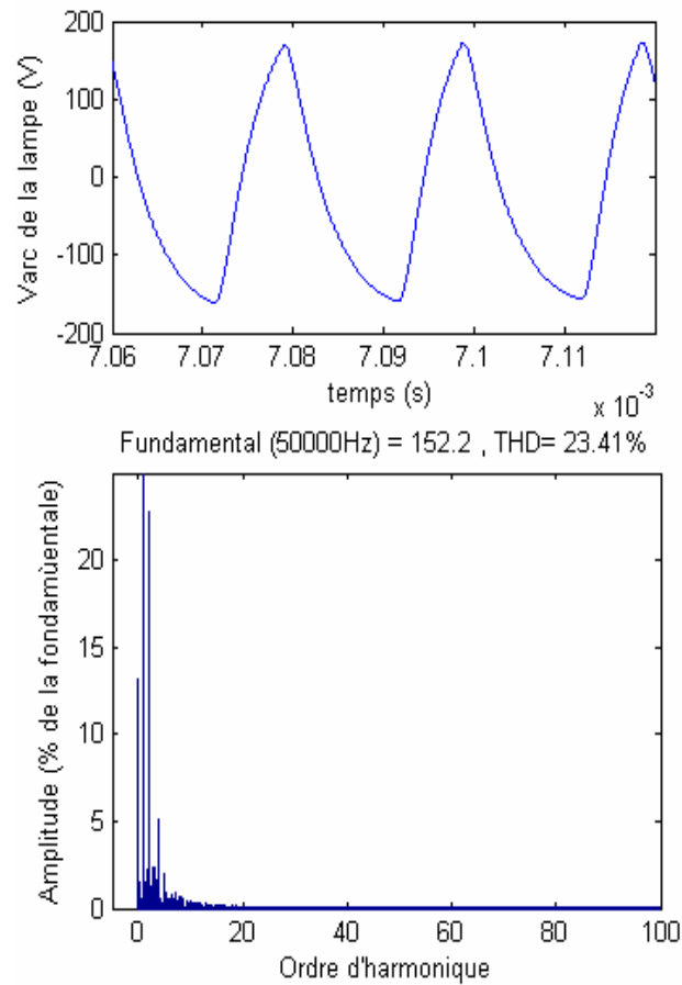
Fig.3.35 : THD de la tension d'arc de la lampe à décharge.
