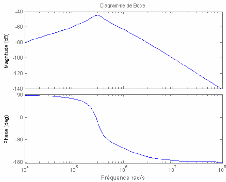
Fig. 4.3 : Diagramme de Bode du système en boucle ouverte.
