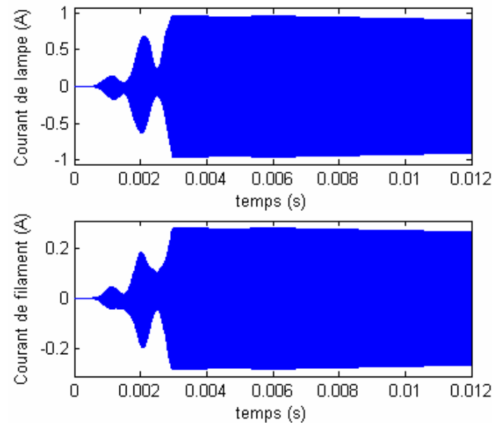
Fig. 4.10 : Courant total et courant de filament de la lampe à décharge.
