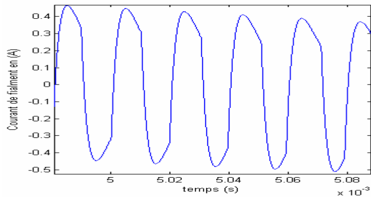
Fig.3.44: Forme d'onde du courant de filament de la lampe à décharge.
