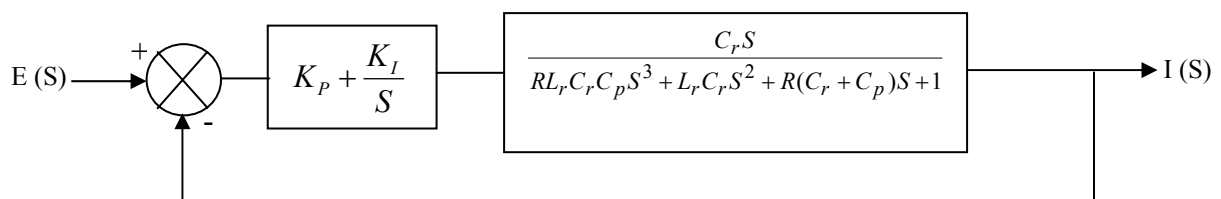
Fig. 4.7: Boucle fermée du système avec régulateur P.I.
