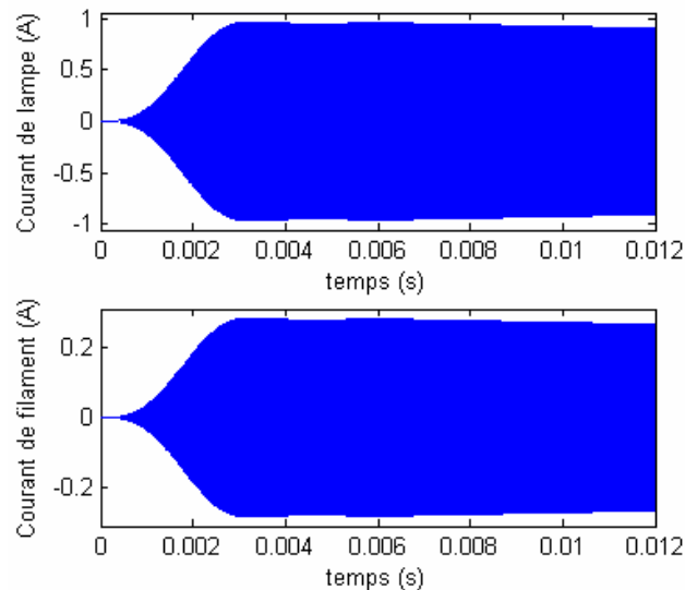
Fig. 5.25: Courant total et courant de filament de la lampe à décharge.
