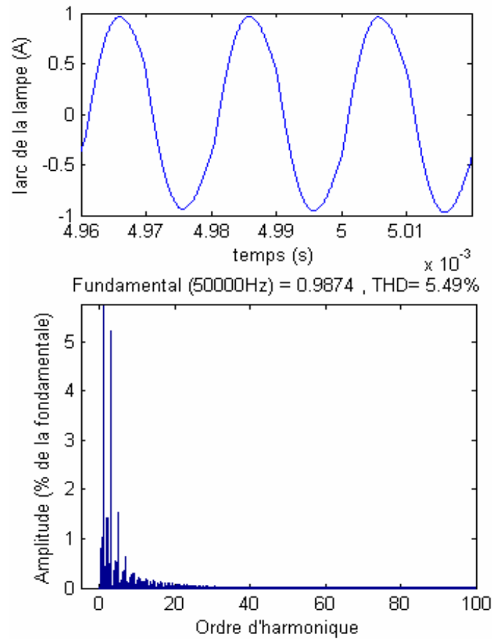
Fig.3.51: THD du courant d'arc de la lampe à décharge.
