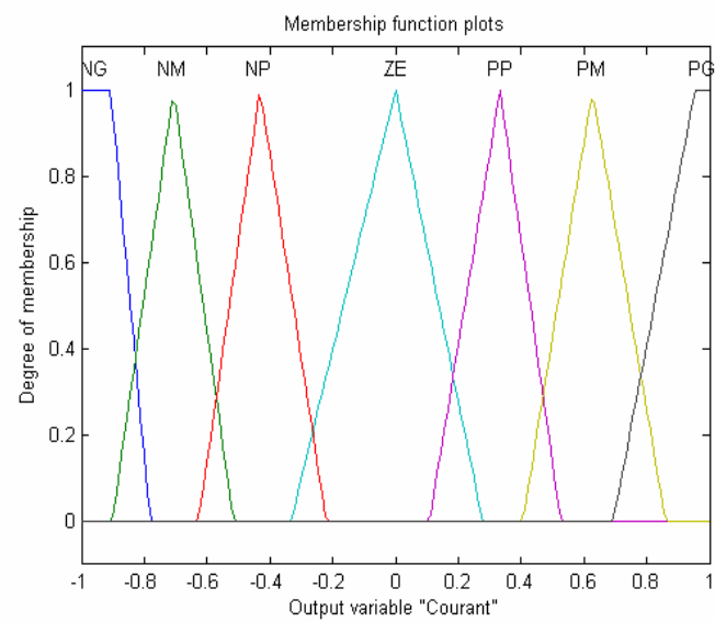
Fig. 5.22 : Fonctions d'appartenance du courant..
