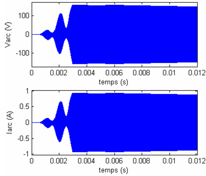
Fig. 4.9 : Tension et courant d'arc de la lampe à décharge.
