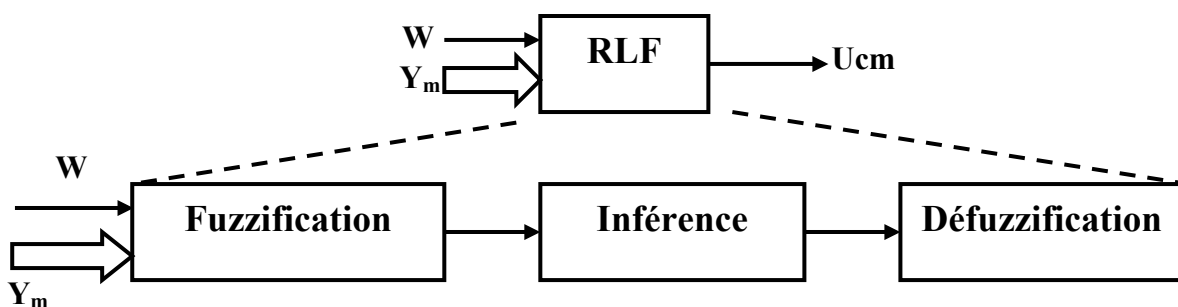
Fig.5.19 : Configuration interne d'un régulateur par logique floue.
