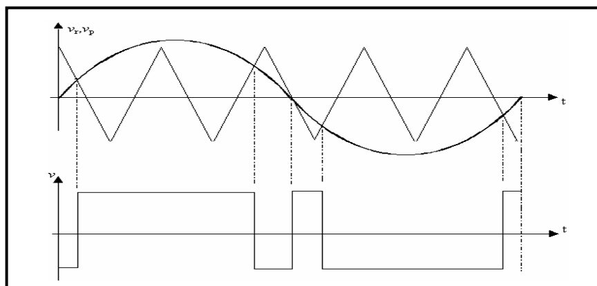
Fig.3.8.b: Surmodulation ( r > 1 ).
