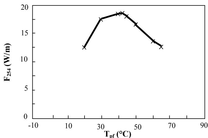
Fig.2.19 : Evolution du flux à 254 nm en fonction de la température du point froid
