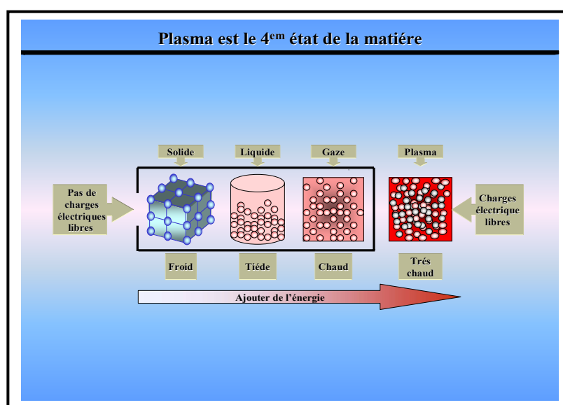
Fig.2.2 : Plasma, 4 ème état de la matière
