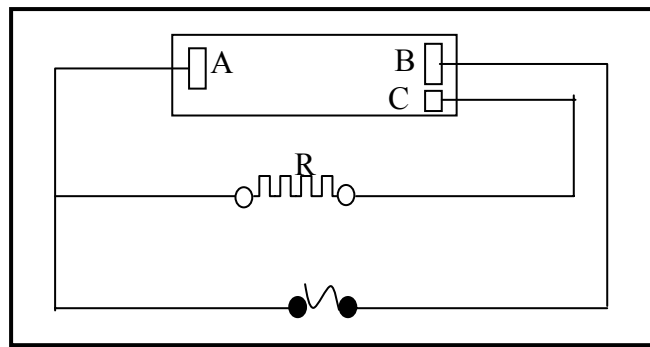
Fig.2.6 : Electrodes auxiliaires
