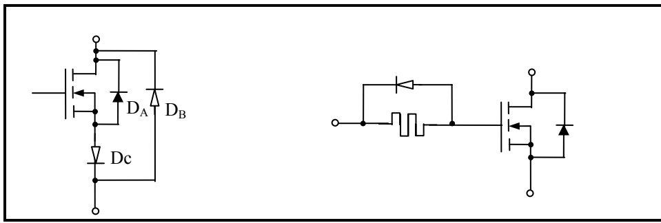
Fig.3.13 : Diode parallèle inverse d'un transistor MOSFET
