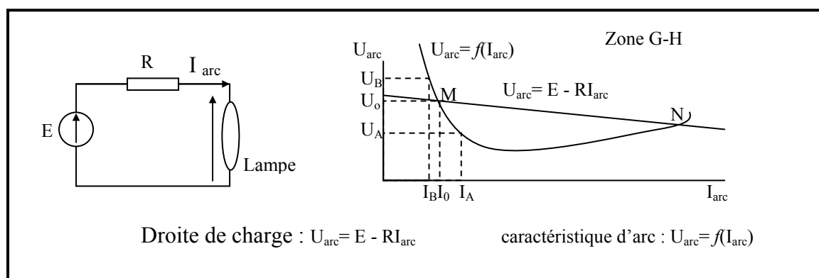
Fig. 2.8 : Montage en source de tension
