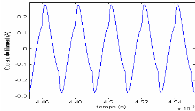
Fig. 5.27: Courant de filament de la lampe à décharge.
