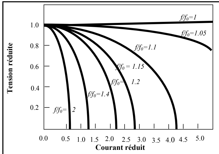
Fig.3.26: Caractéristiques de sortie de l'onduleur en demi-pont.
