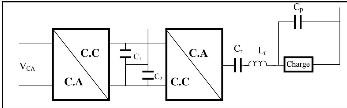
Fig.3.1 : Diagramme block d'un ballast électronique constitué d'un onduleur en demi-pont.
