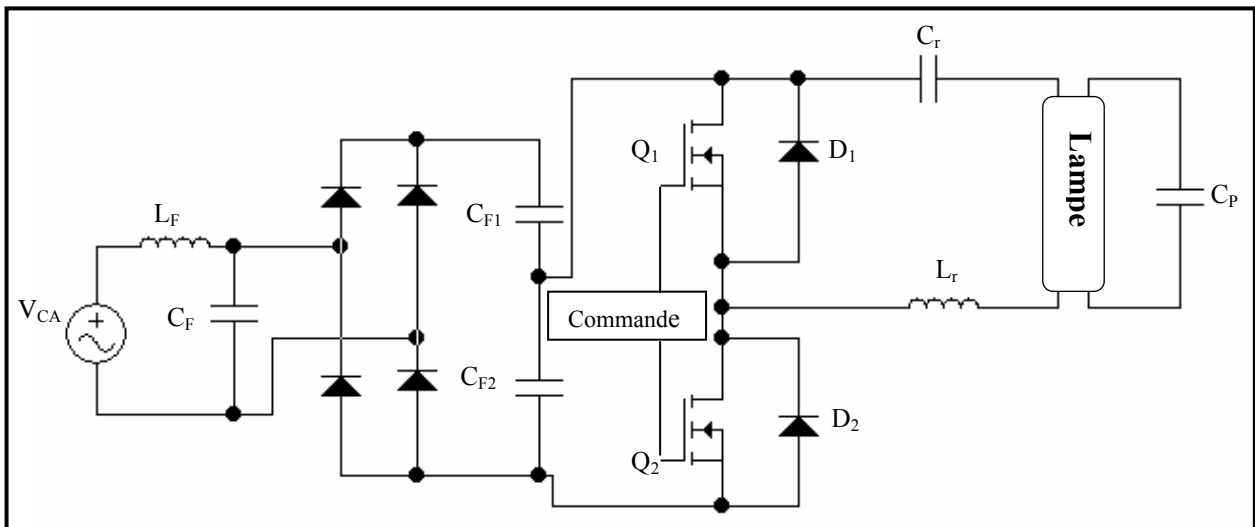
Fig. 3.21: Ballast électronique conventionnel.
