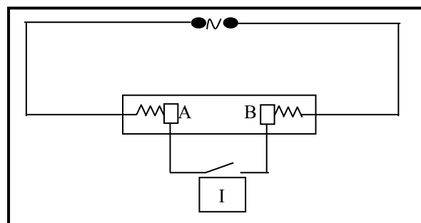
Fig.2.7 : Chauffage préalable des électrodes
