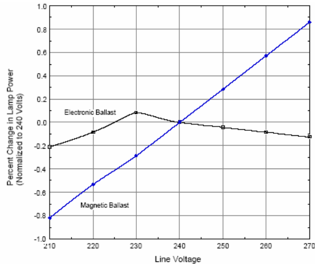
Fig.B-2 : Régulation de la ligne des ballasts électronique et magnétique.
