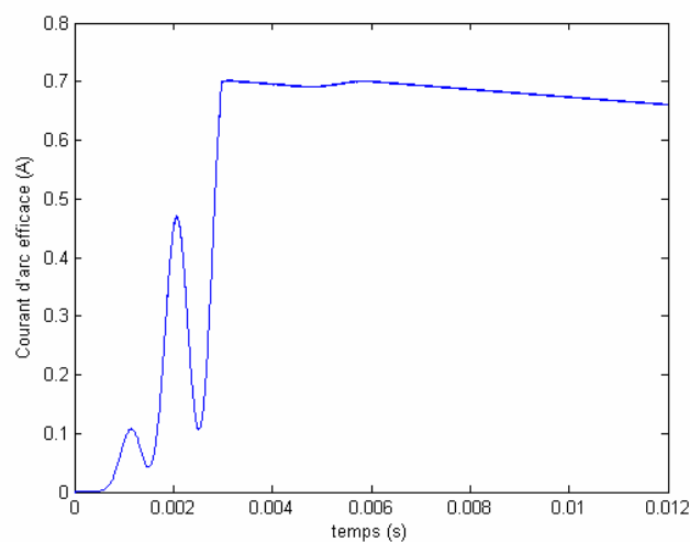
Fig. 4.11: Courant d'arc efficace de la lampe à décharge.
