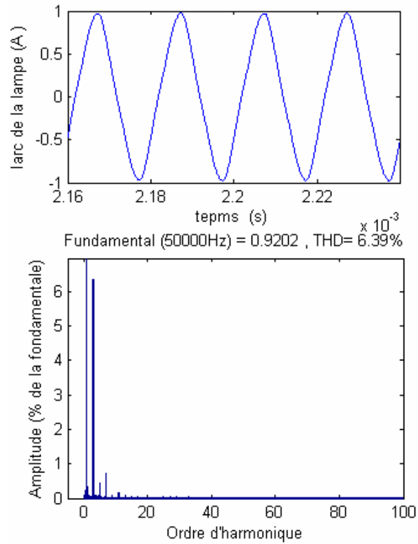
Fig.3.31: THD du courant d'arc de la lampe à décharge.
