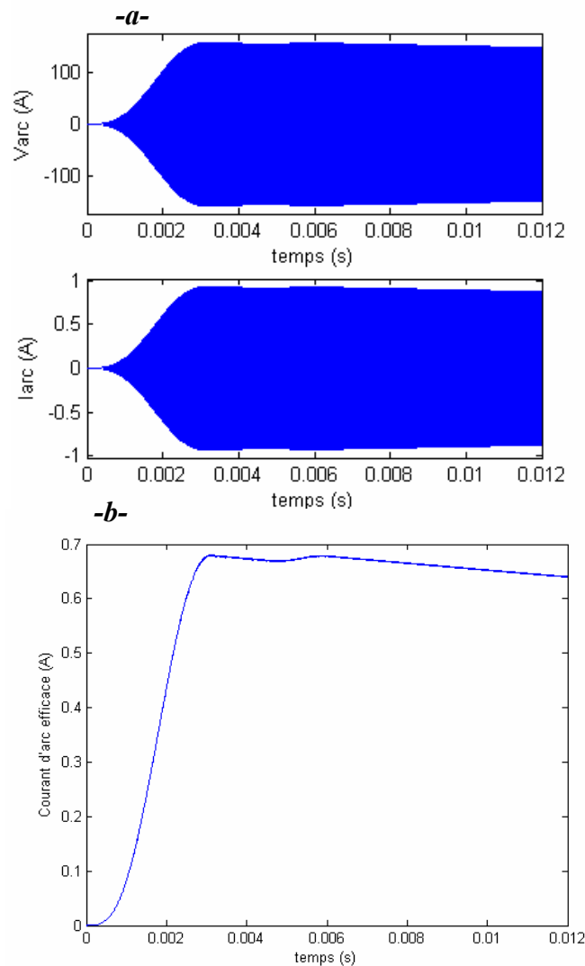
Fig. 5.32 : Forme d'ondes obtenu en appliquant des perturbations de 60%.
