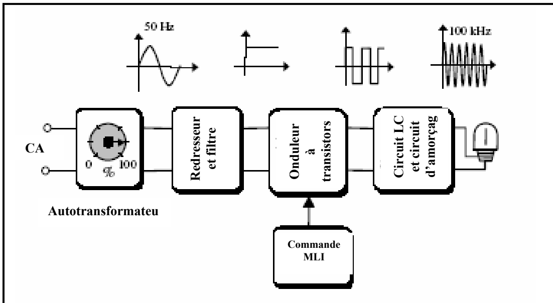
Fig.3.3 : Schéma bloc de l'alimentation.
