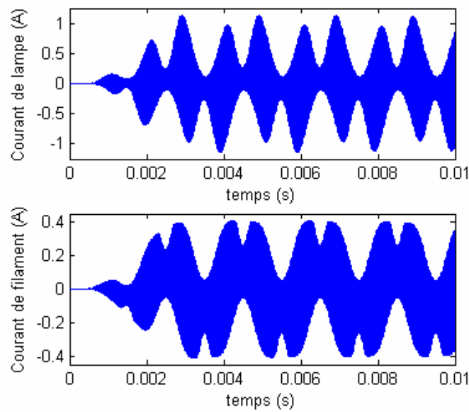
Fig.3.38: Courant total et courant de filament de la lampe à décharge.
