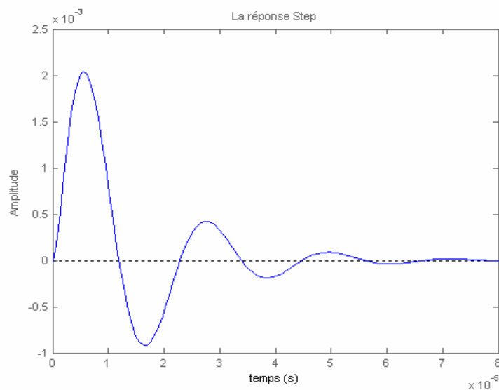
Fig. 4.4 : Réponse indicielle du système en boucle ouverte.
