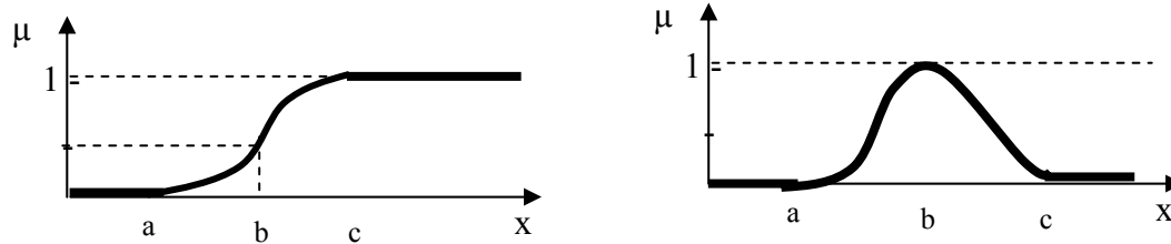
Fig.5.3 : Forme des fonctions d'appartenance.
