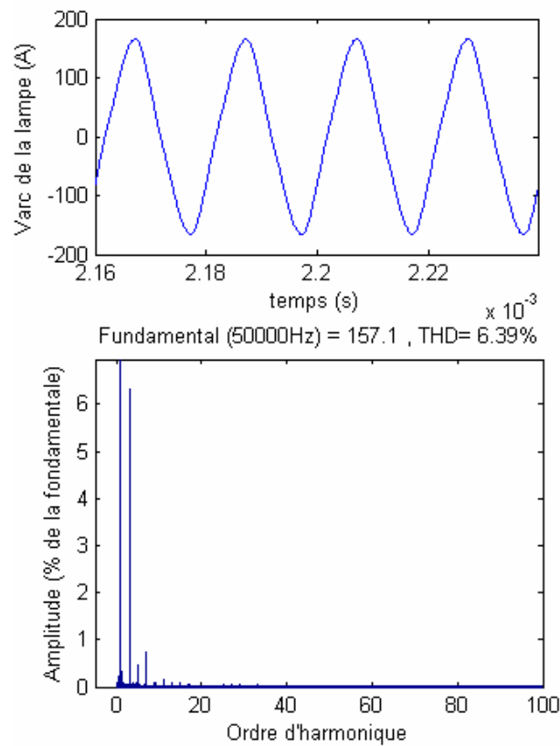
Fig.3.30 : THD de la tension d'arc de la lampe à décharge.
