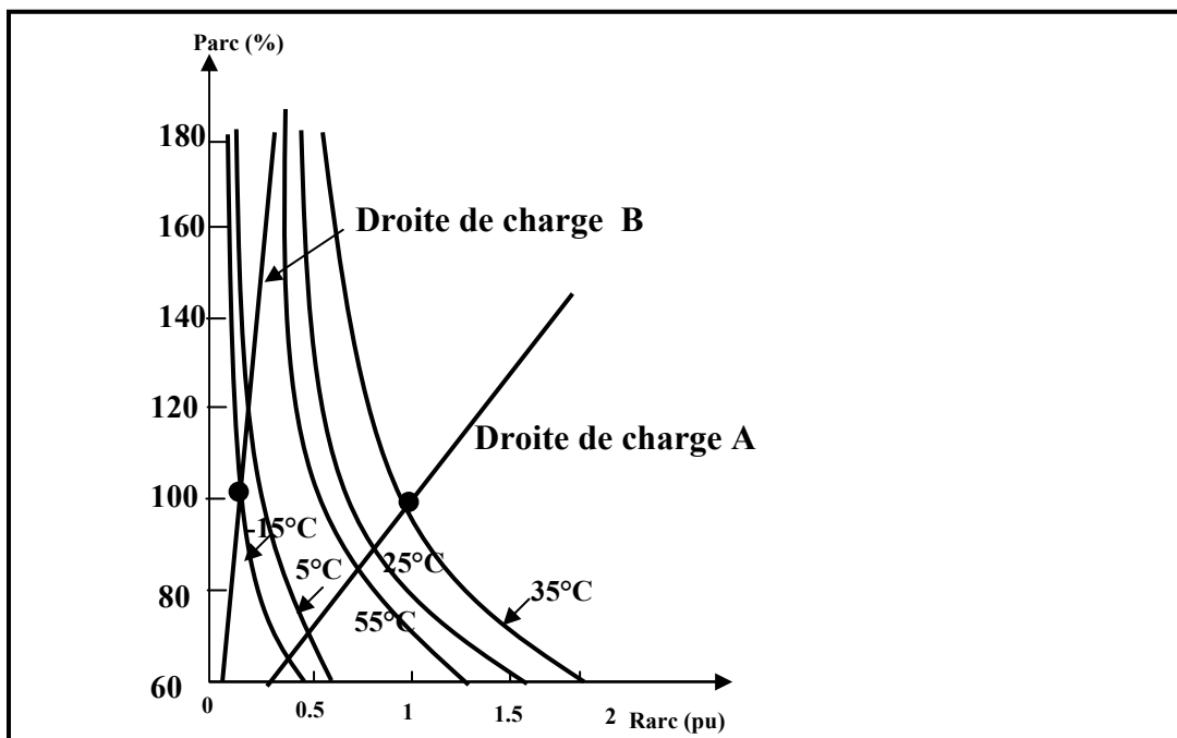
Fig.3.23 : Effets de la température sur la puissance de la lampe.
