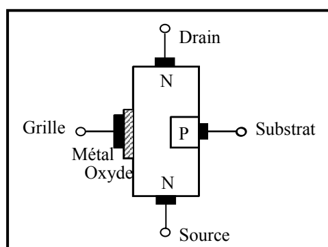
Fig.3.12 : Elements d'un TEC à grille isolée.
