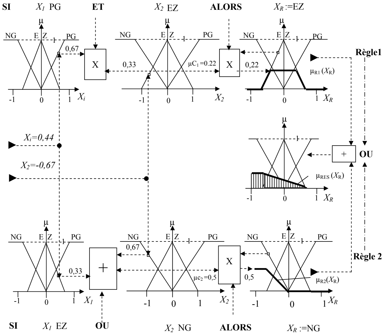
Fig.5.14: Méthode du sum-prod.
