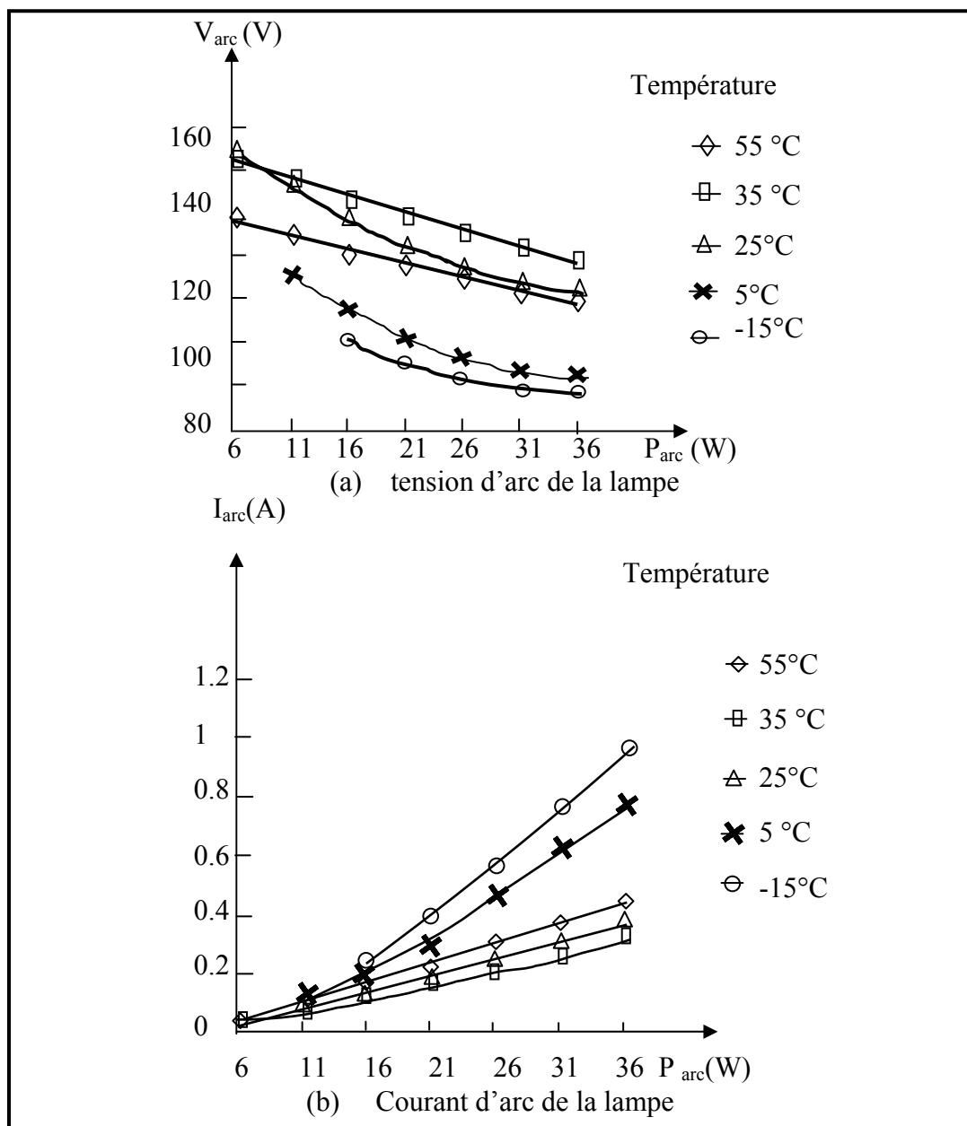
Fig.3.22: Les variations du courant et de la tension de lampe en fonction de sa puissance et de sa température [62].
