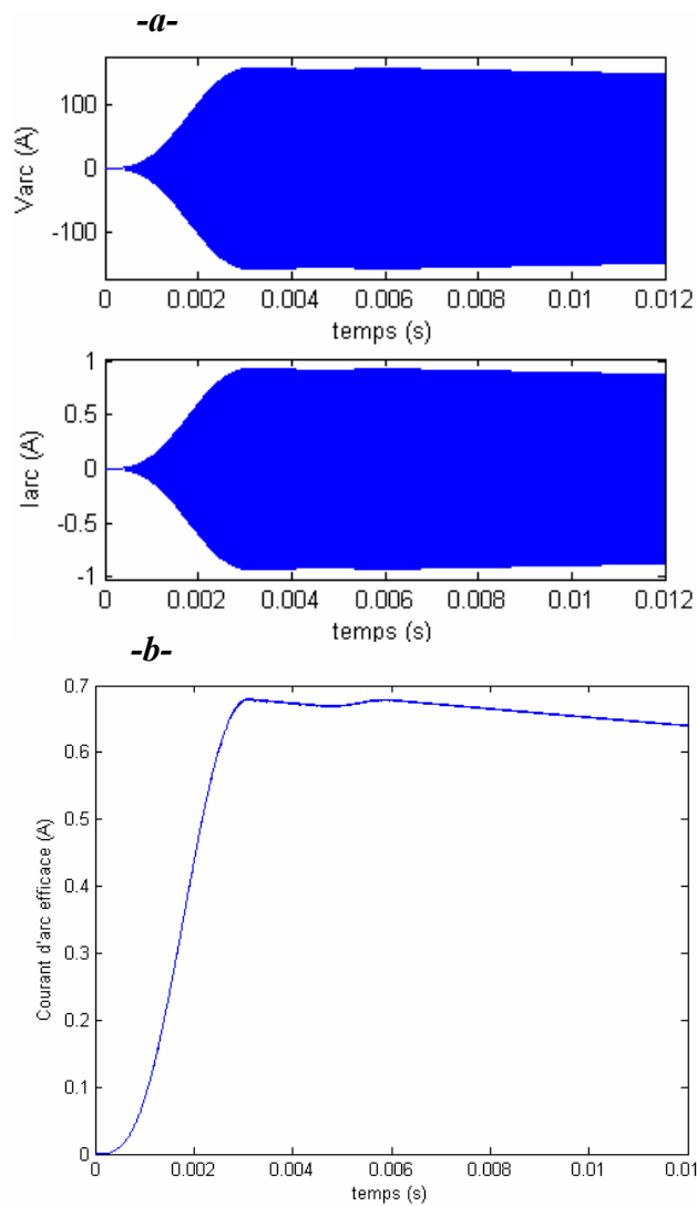
Fig. 5.31 : Forme d'ondes obtenu en appliquant des perturbations de 40%.
