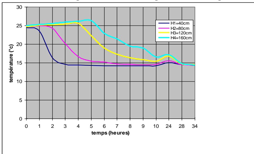
Figure V.5: Plancher entièrement perforé: Évolution de la température dans le temps à 50cm de la paroi
