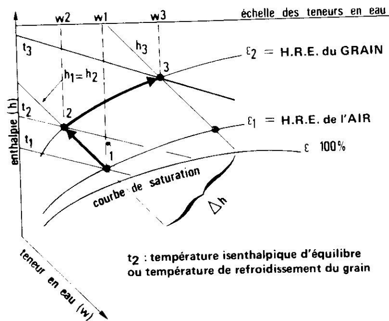
Figure II.12 : Evolution du point caractéristique de l'air sur le diagramme de l'air humide [21].
