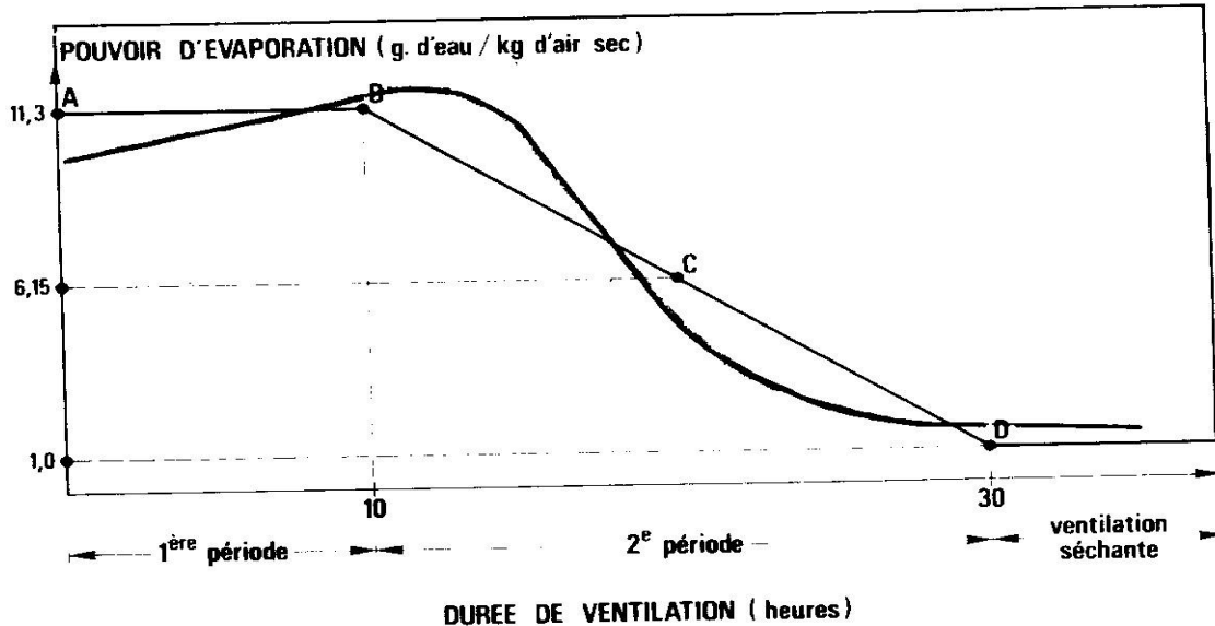
Figure I.3 : Evolution du pouvoir d'évaporation de l'air en fonction de la durée de ventilation [5]
