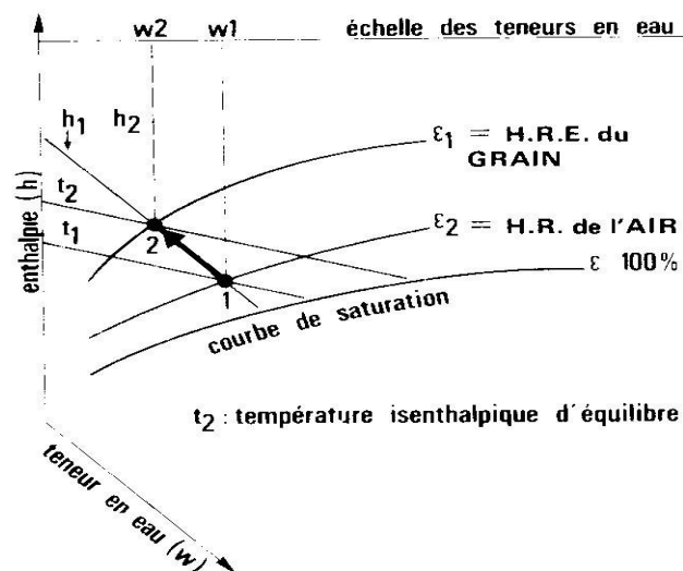
Figure II.10 : Réhumidification de type isenthalpique [21].
