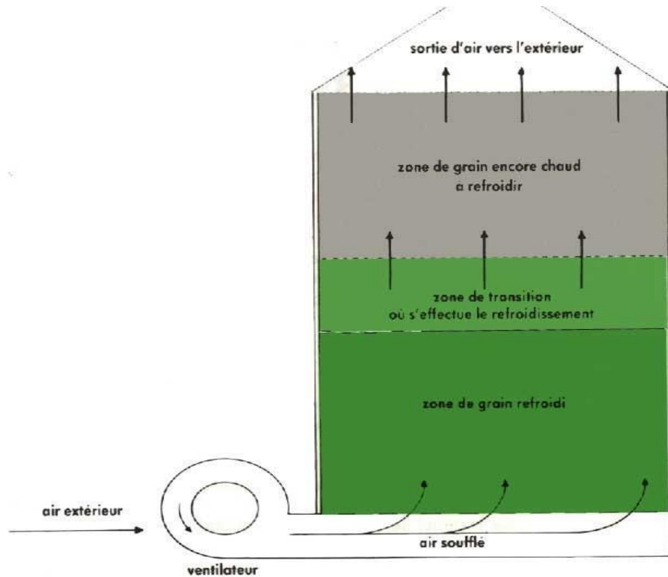
Figure V. 12 : Progression d'une zone de transition dans la masse de grain.
