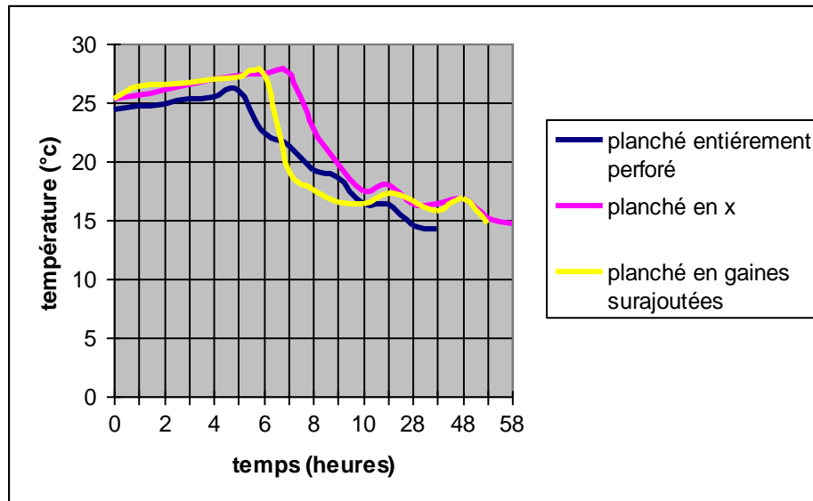
Figure V.22 : Evolution de la température à 10cm de la paroi et à une hauteur de 1,60m de grain pour les trois planchers.
