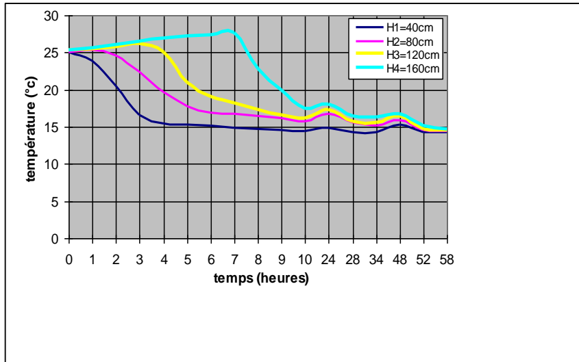
Figure V.6: Plancher en X: Évolution de la température dans le temps à 10cm de la paroi
