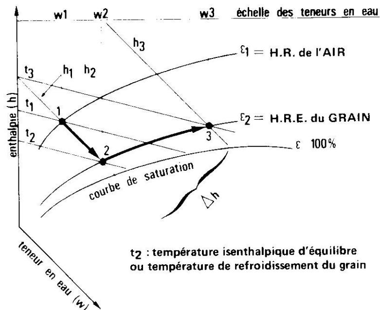
Figure II.11 : Evolution du point caractéristique de l'air sur le diagramme de l'air humide au cours d'une ventilation, avec de l'air dont l' H.R est inférieure à l'H.RE. [21].
