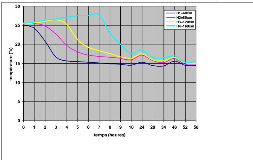
Figure V.7: Plancher en X: Évolution de la température dans le temps à 30cm de la paroi
