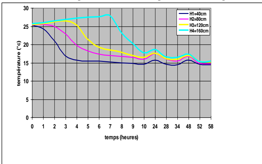
Figure V.8 : Plancher en X: Évolution de la température dans le temps à 50cm de la paroi
