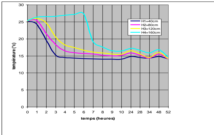
Figure V.9 : Plancher en gaine surajouté: Évolution de la température dans le temps à 10cm de la paroi
